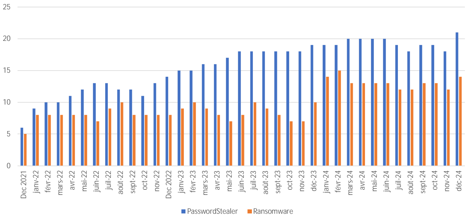
Evolution de la part des PasswordStealer et Ransomware
